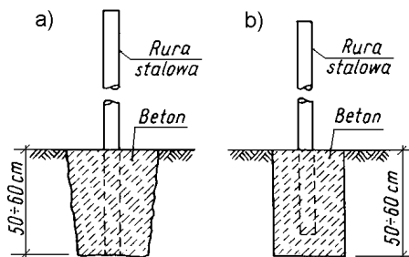
Rys. 4. Przykład ustawiania słupków ogrodzenia (wg [6])
