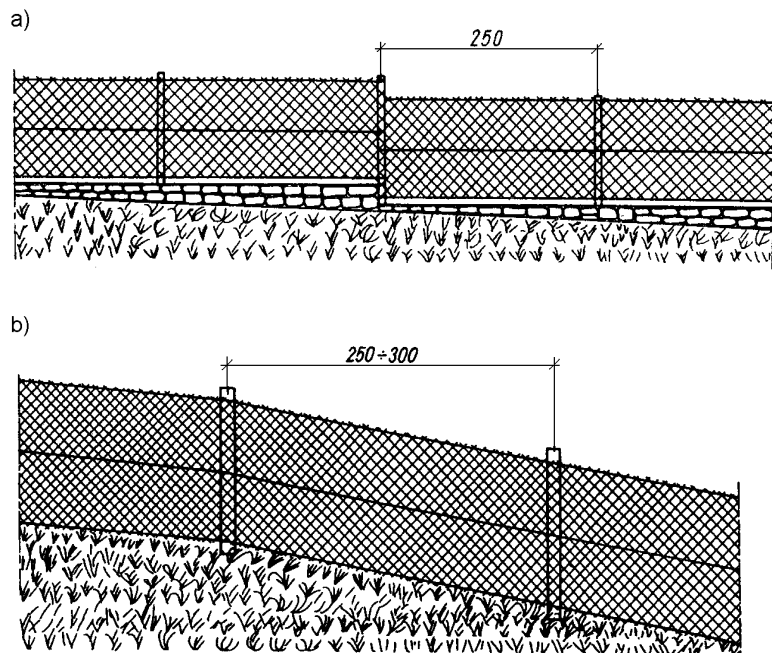
Rys. 6. Przykład ustawienia ogrodzenia siatkowego na terenie pochyłym (wg [6]) 4. Ogrodzenie ze stopniami wysokości 25÷30 cm (przy spadku terenu od 1:16 do 1:30) 5. Ogrodzenie równoległe do terenu
